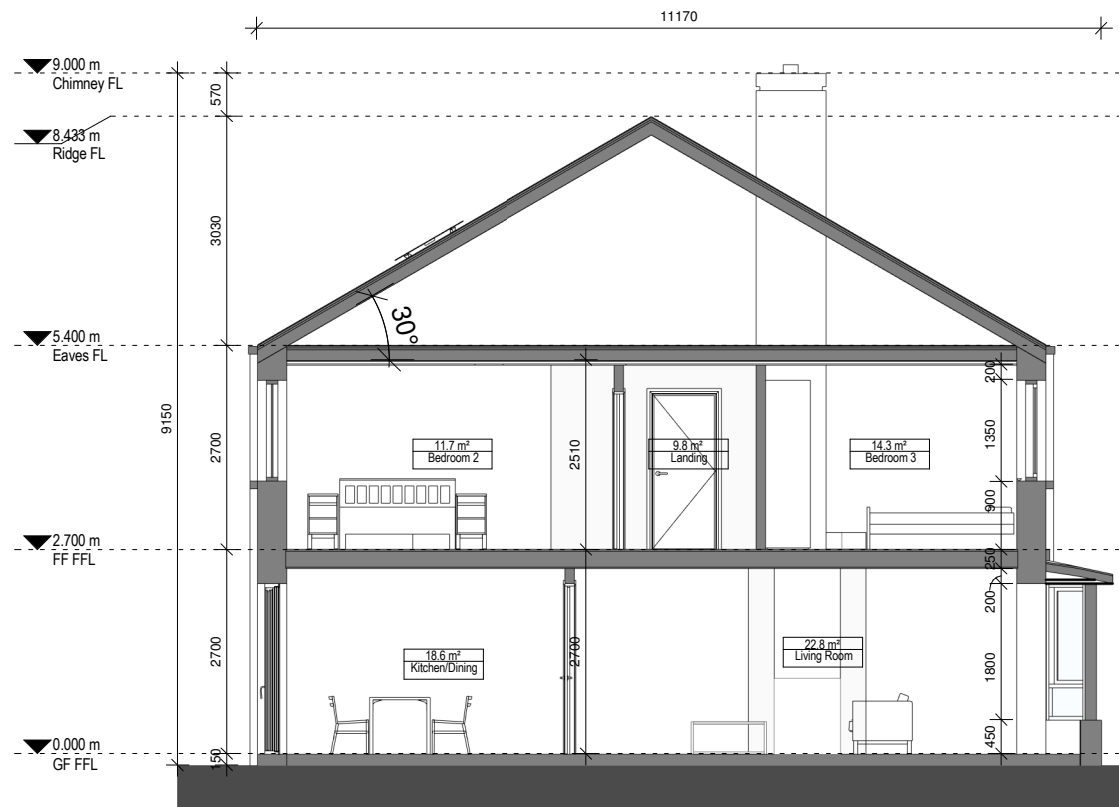
1 Section 1 1:100 @ A3
